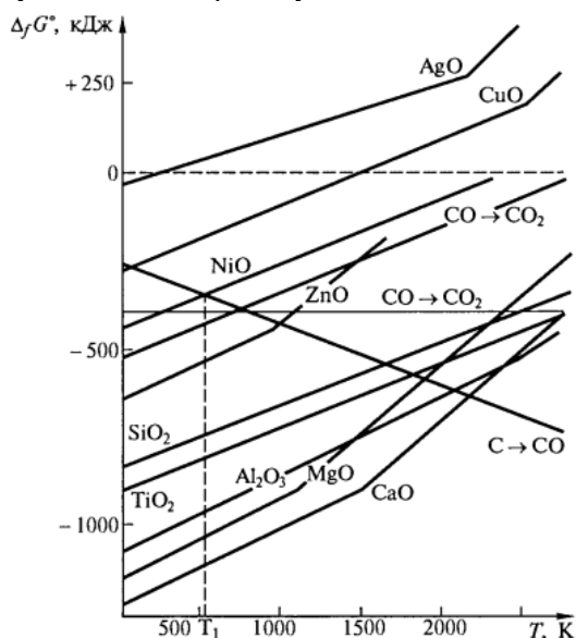
Пример диаграммы Эллингама для восстановления оксидов металлов
